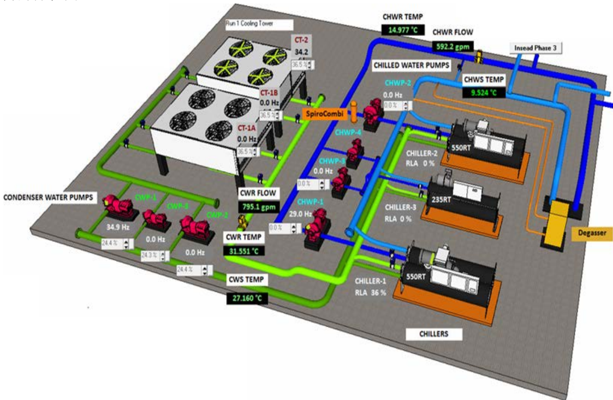
图 1. 中央空调系统的基本结构示意图
