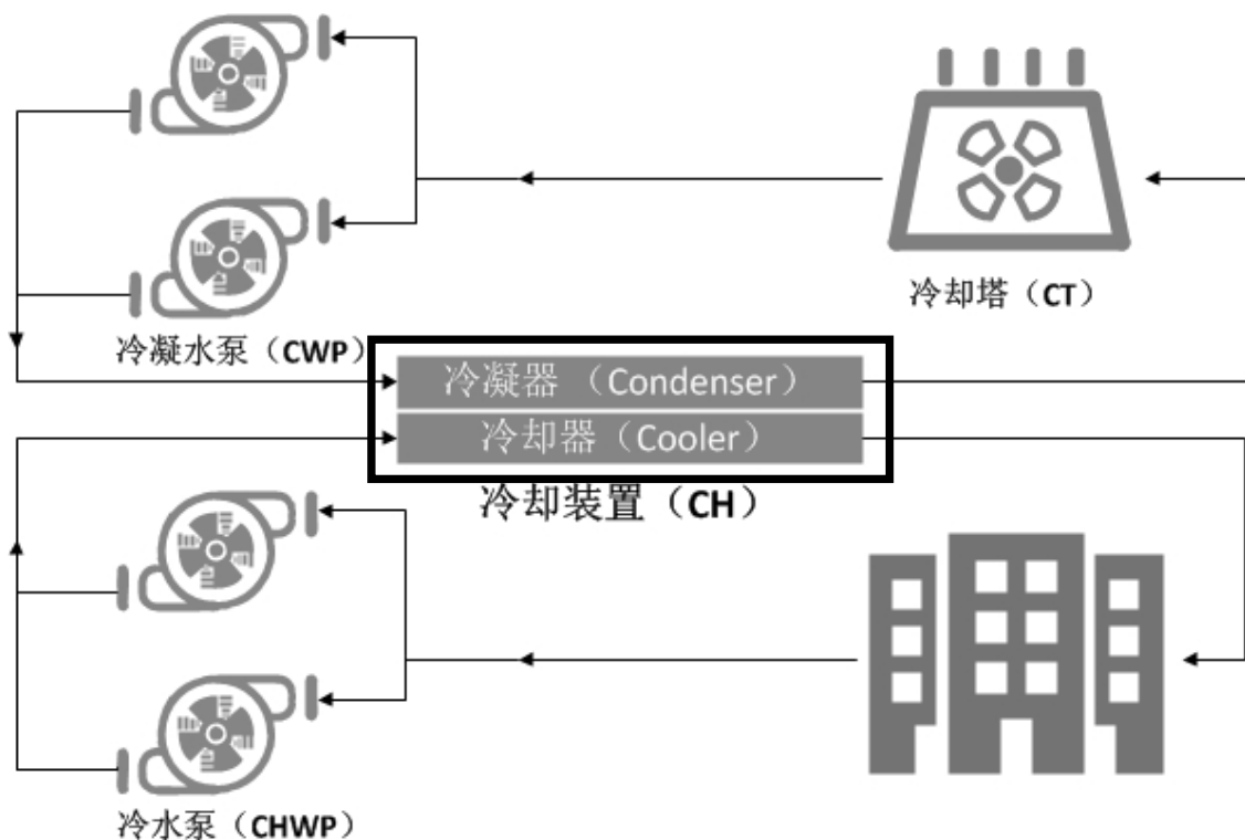
图2. 中央空调系统的工作原理图。
